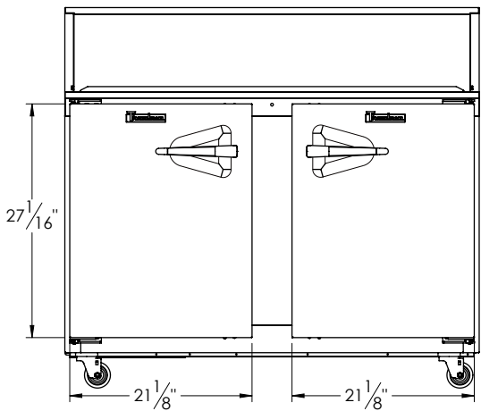
ELEVATION
